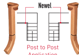
Left-hand 2 Riser No Cap Right-hand 2 Riser No Cap
